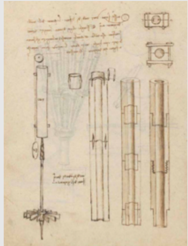
Figura 7. Fabricación de tubos y conexiones de madera. (Contreras, 2015)
